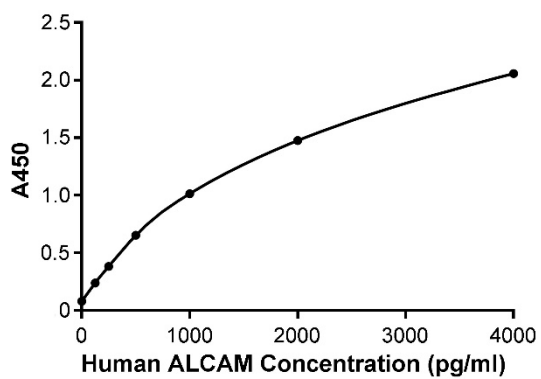
图3. Human ALCAM ELISA Kit的标准曲线。实测数据会因实验条件、检测仪器等的不同而存在差异，图中数据仅供参考。
